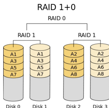
Фигура 3. RAID 1+0
