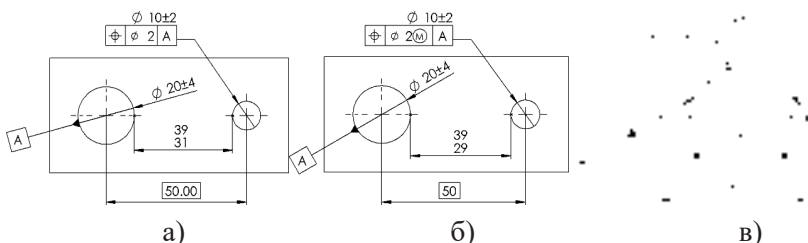
Фигура 2. Размерен анализ на детайл с геометрични допуски
