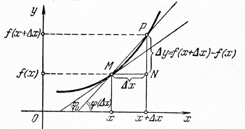
Фигура 2. Графично изображение на y=f(x) декартова координатна система
