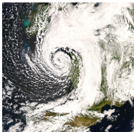
Фигура 6. Сателитна снимка на циклон над Европа според: http://www.weather.com/
