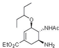
3. Oseltamivir
