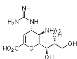
4. Zanamivir
