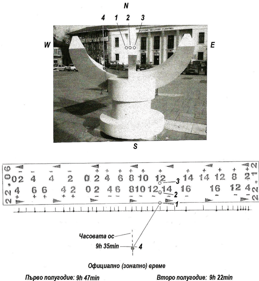
Фиг. 4. Определяне на официалното (зонално) време
