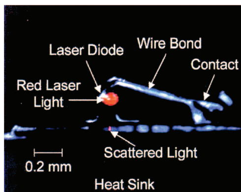
Фиг. 2. Полупроводниковият лазер на екипа на Nick Holonyak 1962 г. (излъчващ във видимата област)
